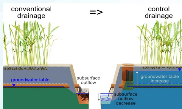
شکل ۳-۱۰- تصویری از یک زهشی کنترل شده و نحوه کارایی آن
