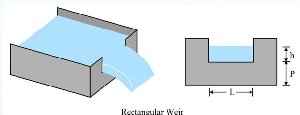
Rectangular Weir شکل ۴-۱- سرریز مستطیلی لبه تیز
