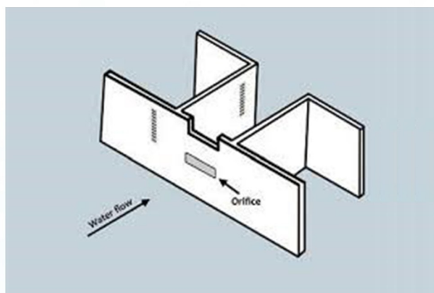
شکل ۴-۳- شکل شماتیک یک روزنه مستطیلی
