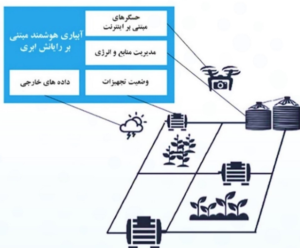
شکل ۲-۲- بخش‌های اساسی آبیاری هوشمند مبتنی بر اینترنت اشیاء و رایانش ابری
