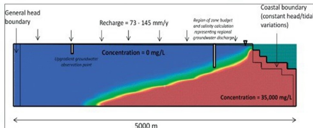
شکل ۵-۴- نمونه‌ای از شبیه‌سازی انجام‌شده در مدل SEAWAT
