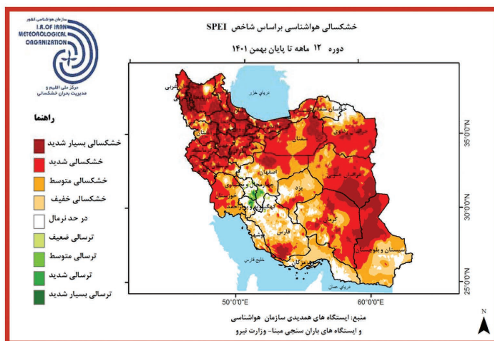
شاخص SPEI دوازده ماهه تا پایان بهمن ماه ۱۴۰۱.
