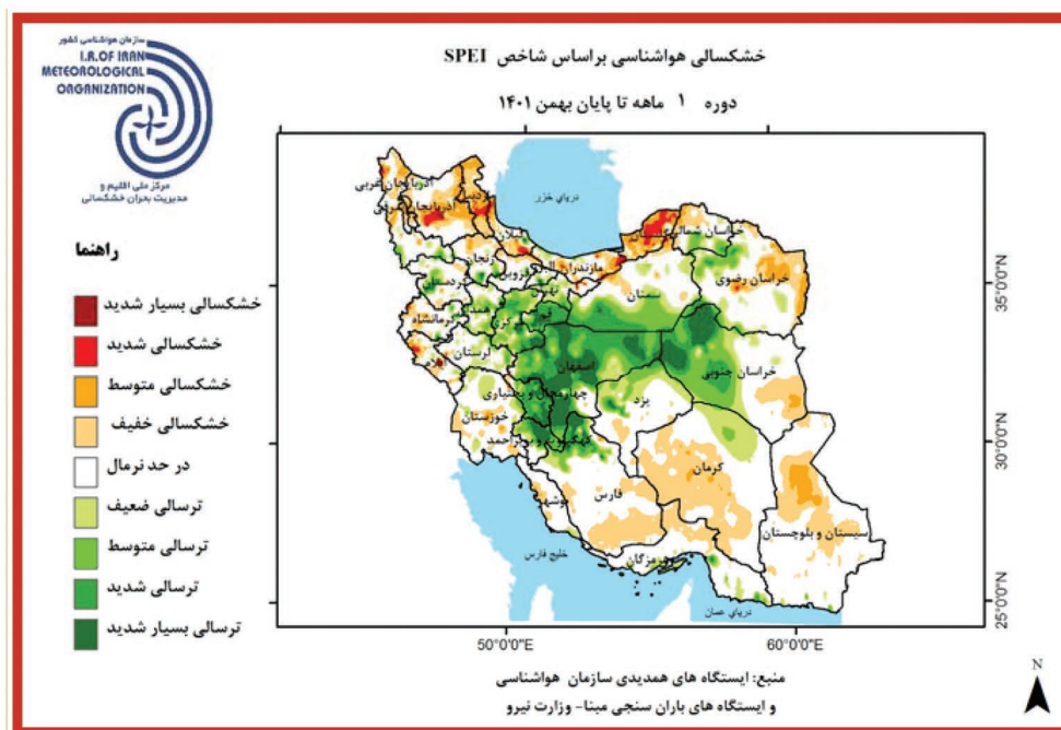
شاخص SPEI یک ماهه بهمن ماه ۱۴۰۱.
