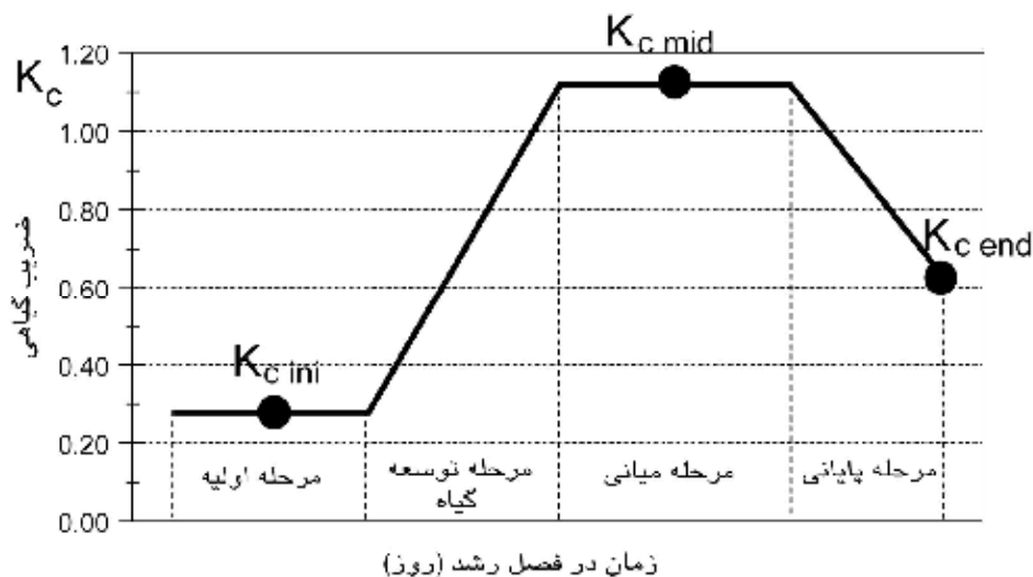
شکل ۳۴- منحنی ضریب گیاهی
