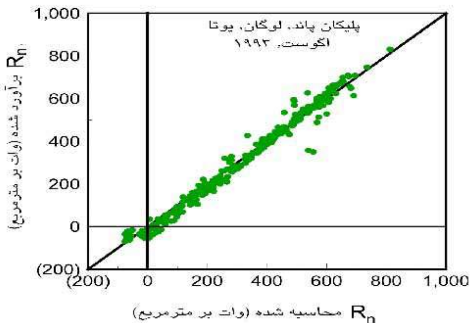
شکل ۵-۳- R_n اندازه‌گیری شده و برآورد شده (در طول دوره ۲۰ دقیقه‌ای) برای نوعی علف (با رشد کامل) در نزدیک لوگان، یوتا (ایالات متحده آمریکا) در ماه اوت سال ۱۹۹۳ (به نقل از آلن و همکاران، ۱۹۹۴).
