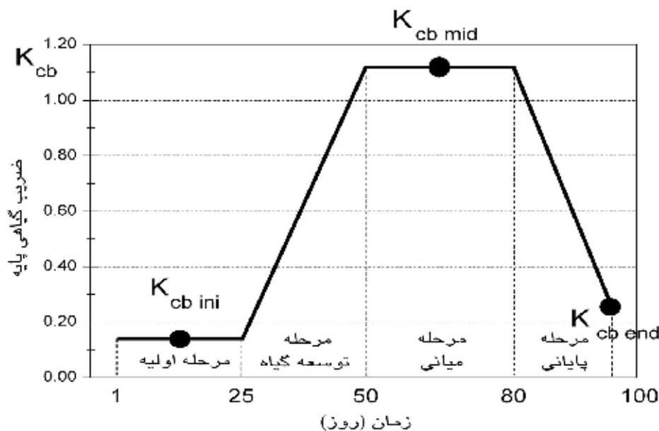
شکل ۳۷- منحنی ضریب گیاهی پایه لوبیا دانه‌ای در چهار مرحله رشد با طول به ترتیب ۲۵، ۲۵، ۳۰ و ۲۰ روز (مثال ۲۹)
